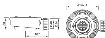
Válvula Ø90 mm com sifão
