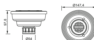
Válvula de descarga vertical
