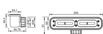
Válvula 265x64 mm com sifão duplo
